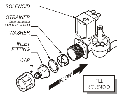
Fig. 15 Fill Solenoid
