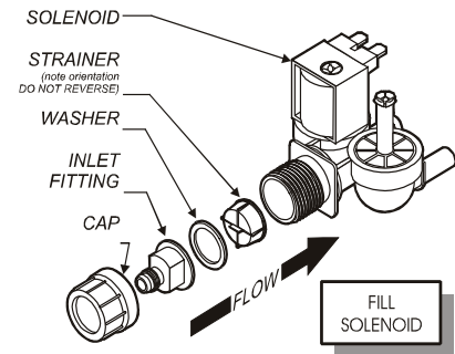
Fig. 15 Fill Solenoid
