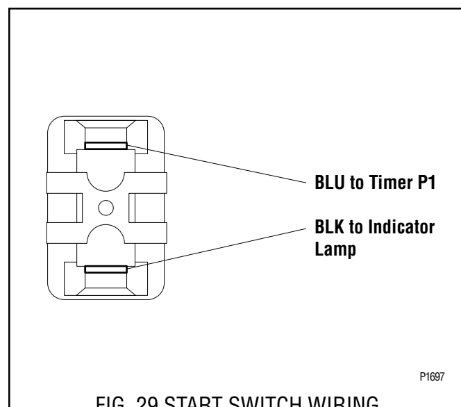
FIG. 29 START SWITCH WIRING
