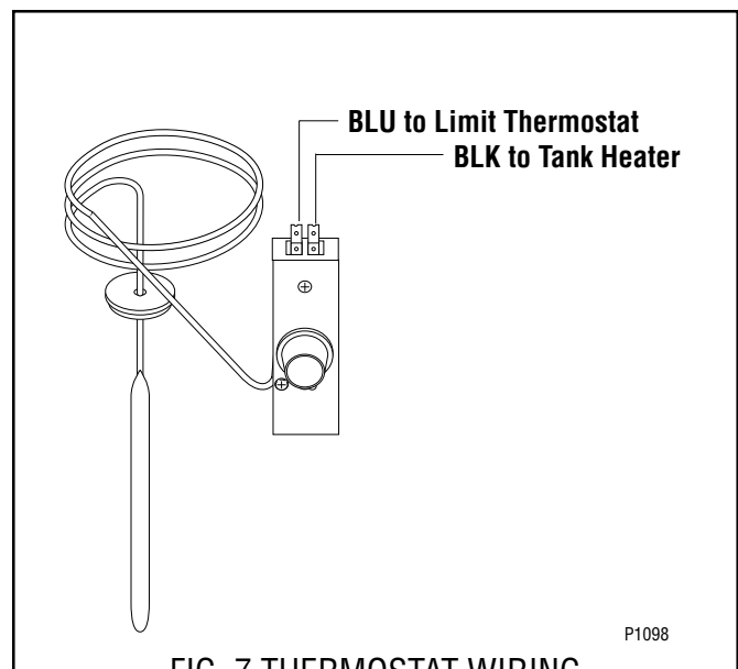
FIG. 7 THERMOSTAT WIRING
