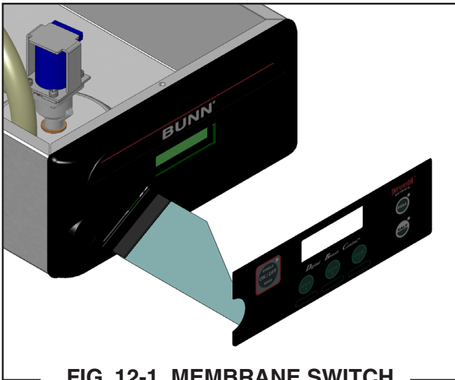
FIG. 12-1 MEMBRANE SWITCH
