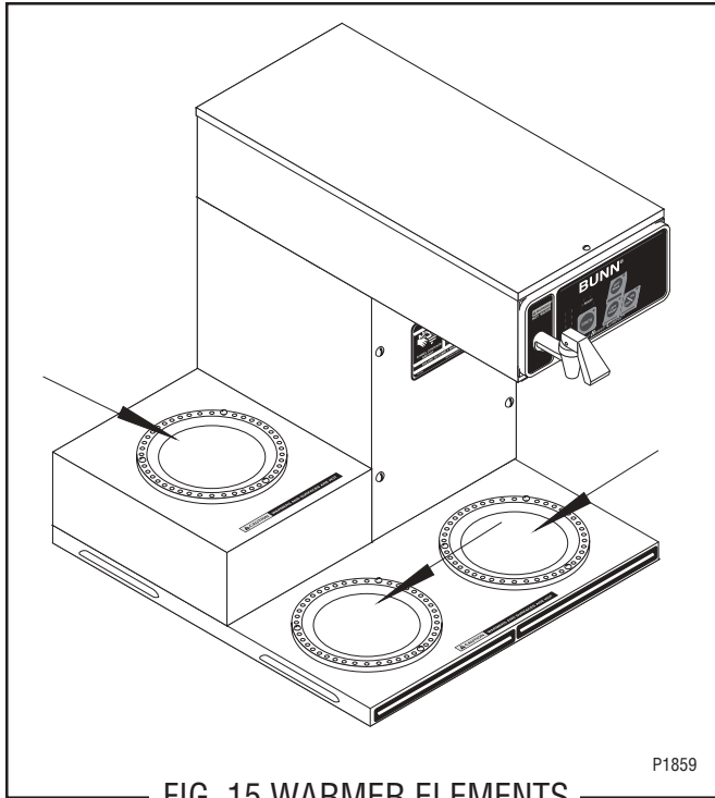
FIG. 15 WARMER ELEMENTS
