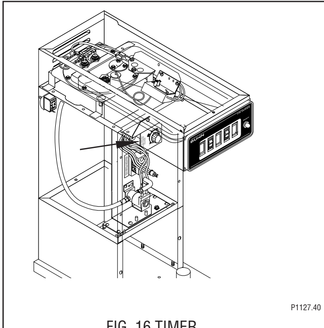
FIG. 16 TIMER
