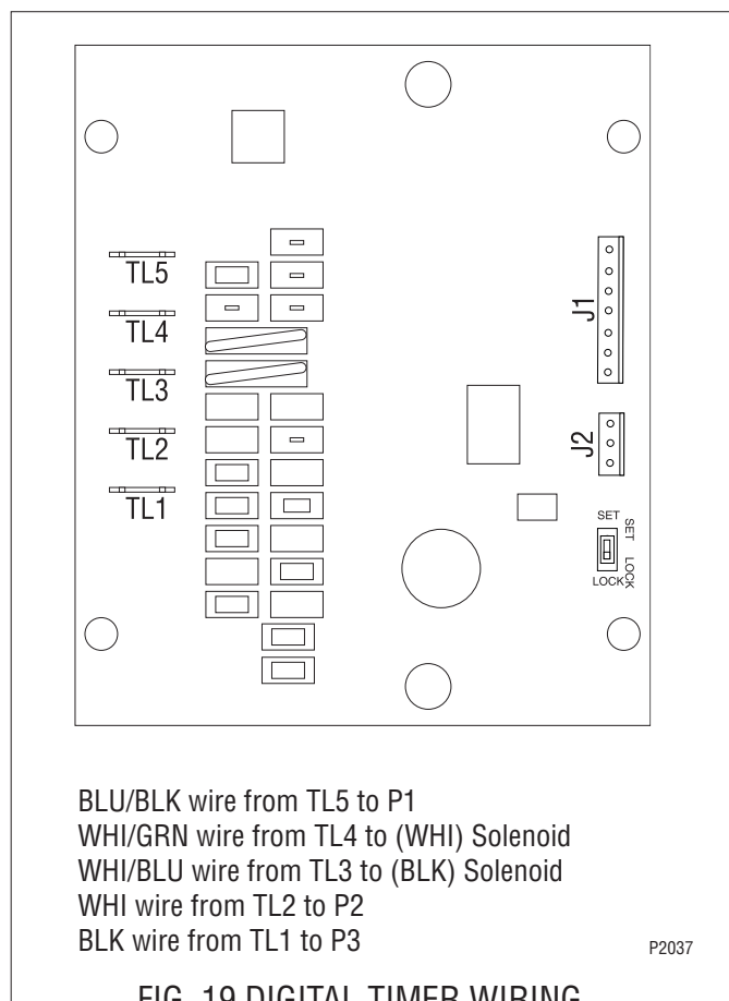
FIG. 19 DIGITAL TIMER WIRING
