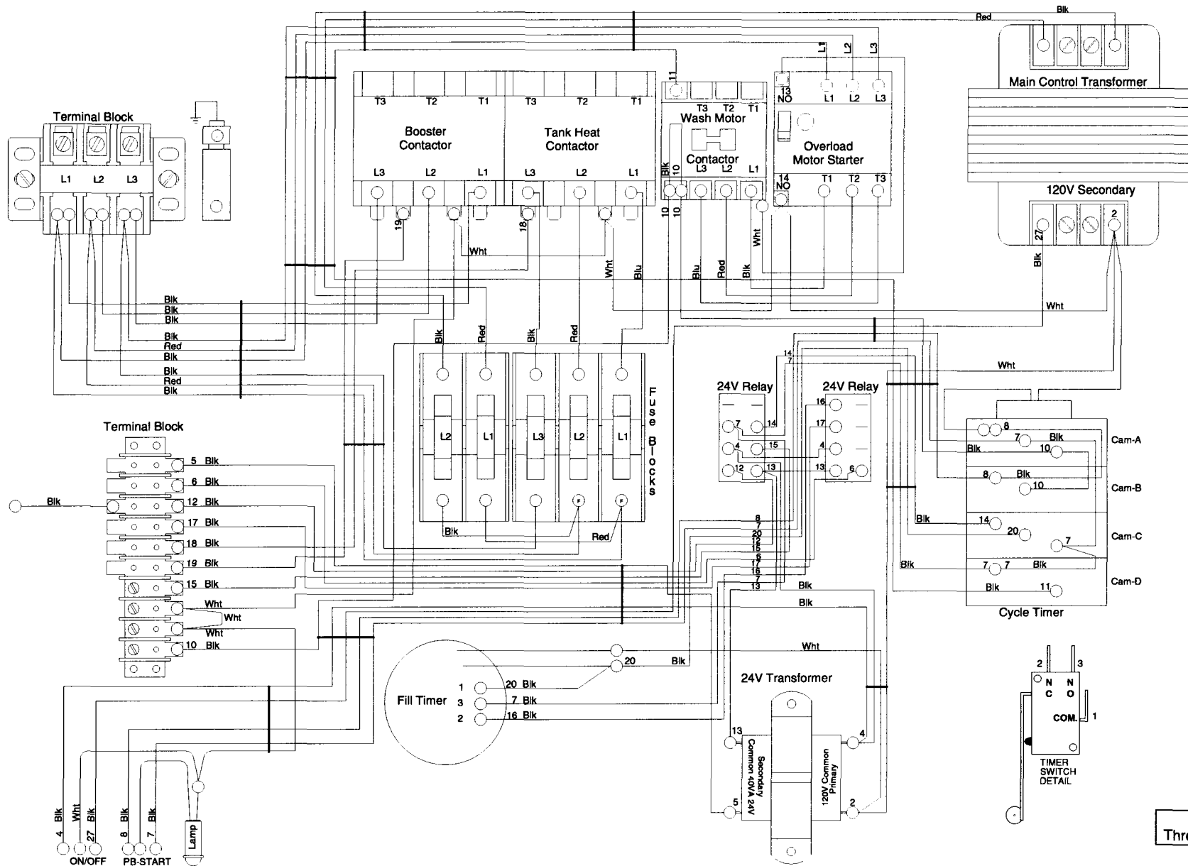
Fig. 38 – Wiring Diagram D-HB, 3 Phase
