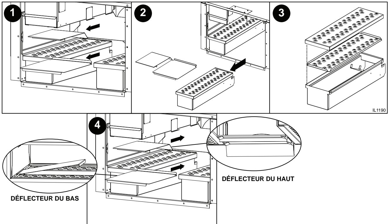
Enlever / Monter les déflecteurs et les doigts
