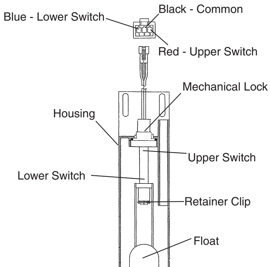
Fig. 1 Float Switch
